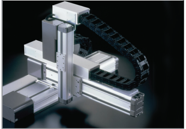
מערכת הנעה תלת צירית ROBOT MODULE תוצרת NSK
