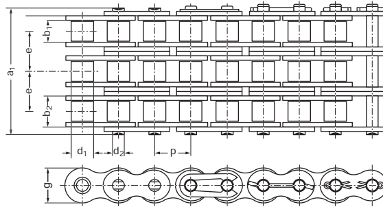
Roller link Pin link מנעול עם קפיץ נעילה מנעול פין פציל
