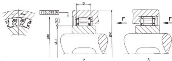
כיוון סיבוב הטבעת החיצונית במבט מכיוון F
