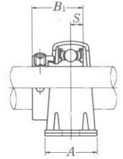
ENPP / AELPP נעילה אקצנטרית
