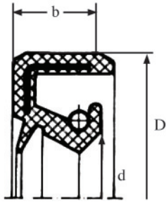
אטימת שפה כפולה TC
