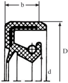
אטימת שפה כפולה דצ
